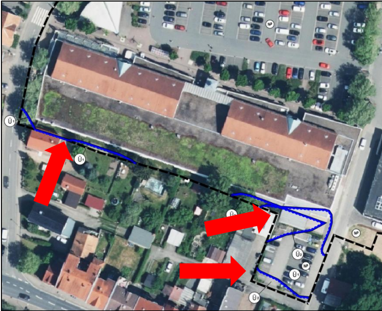
Abbildung 15: Grenze Überschwemmungsgebiete – nachrichtliche Übernahme gem. § 9 (6) BauGB (Quelle: Ausschnitt aus Bebauungsplan)
