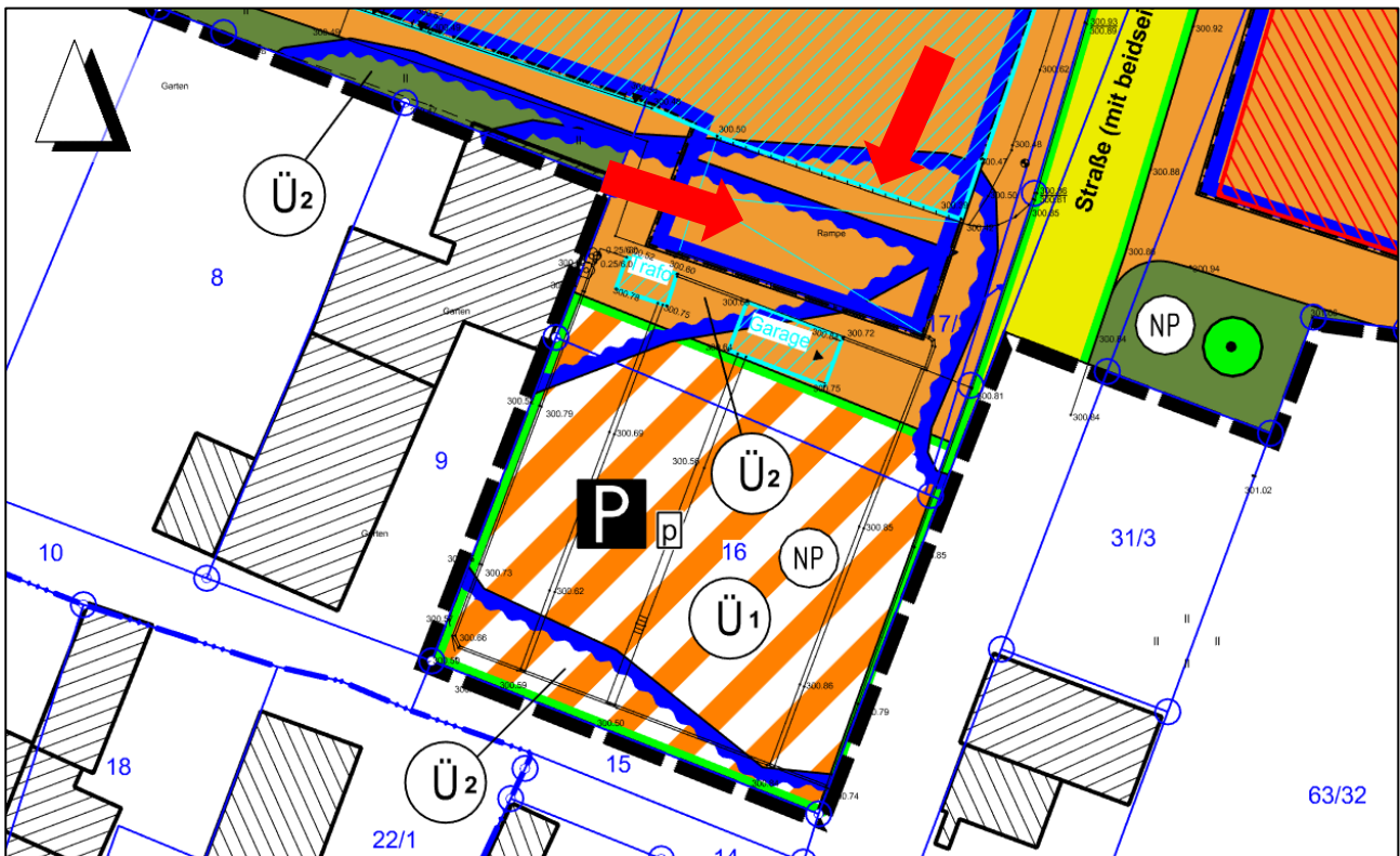
Abbildung 12.2: von Überschwemmungsgebieten betroffene Rampe und Teilbereich des Einkaufszentrums (rote Pfeile; Quelle: Ausschnitt aus Bebauungsplan)
